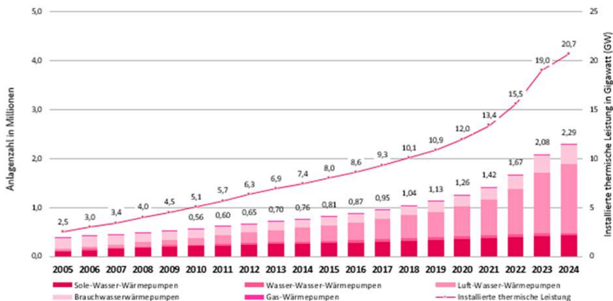
Abbildung 20: Entwicklung des Wärmepumpenbestandes in Deutschland
