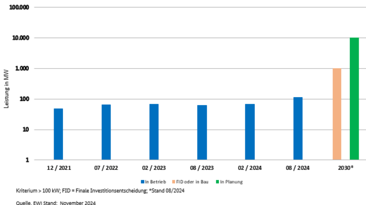
Abbildung 16: Entwicklung der installierten Leistung von Elektrolyseuren
