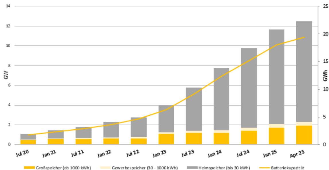
Abbildung 15: Installierte Batterieleistung und Gesamtkapazität gemäß Marktstammdatenregister
