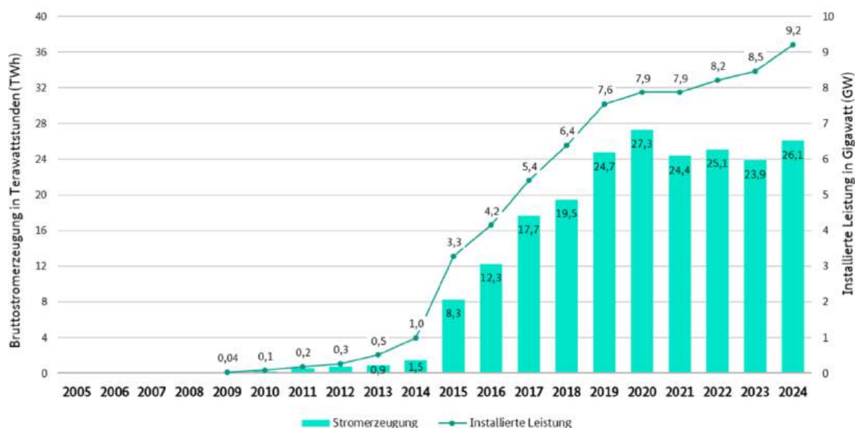
Abbildung 9: Bruttostromerzeugung und installierte Leistung Wind auf See
