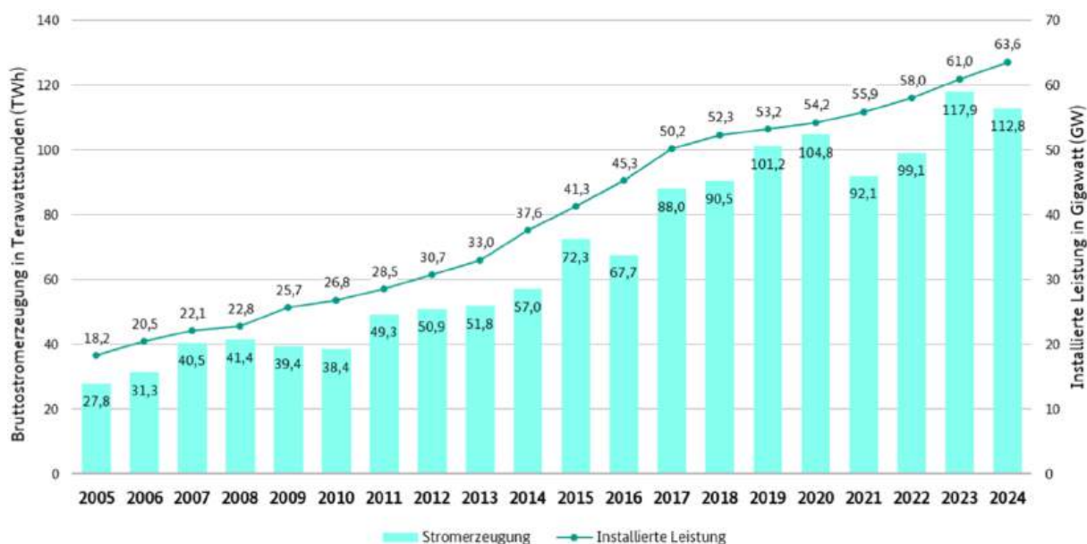
Abbildung 8: Bruttostromerzeugung und installierte Leistung Wind an Land
