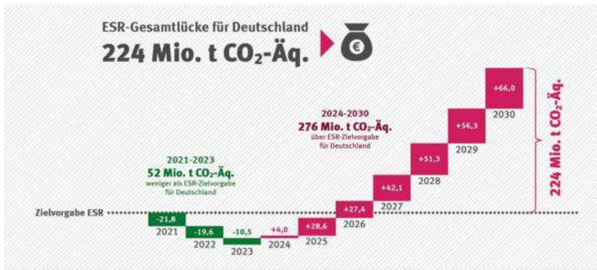
Abbildung 4: ESR-Emissionen Deutschlands zwischen 2021 und 2030 sowie Gesamtlücke nach Projektionsdaten 2025
