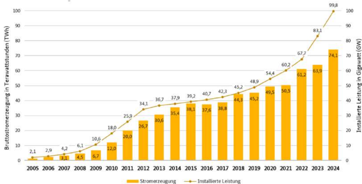
Abbildung 7: Bruttostromerzeugung und installierte Leistung Photovoltaik
