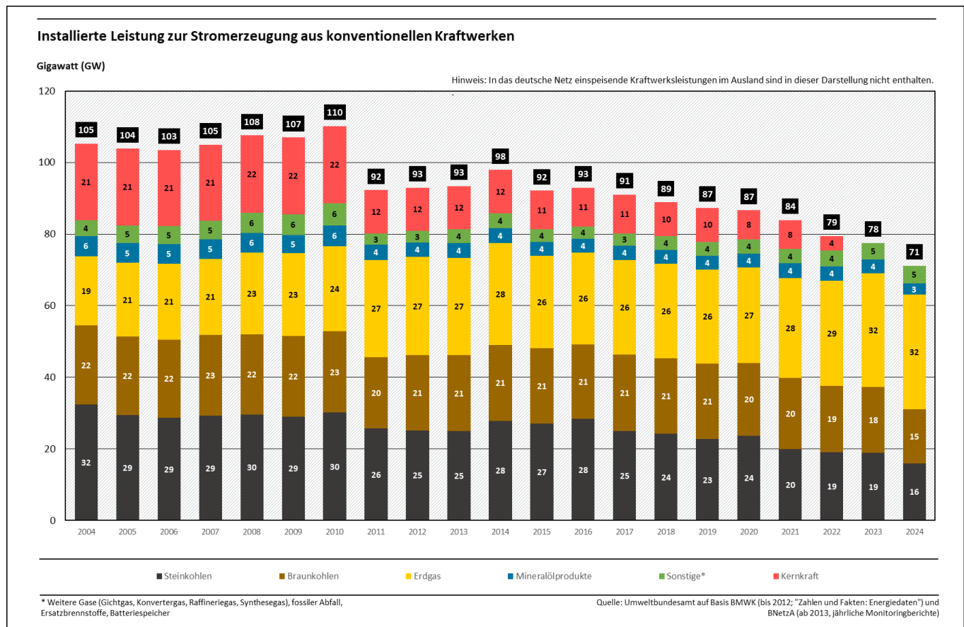
Abbildung 12: Entwicklung der installierten elektrischen Leistung von Kraftwerken ab 10 Megawatt aus fossilen Energien
