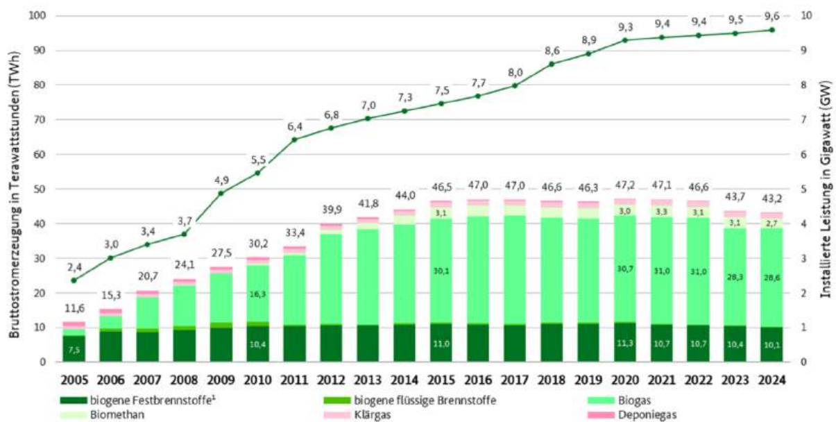
Abbildung 10: Entwicklung der Bruttostromerzeugung und installierten Leistung von Biomasseanlagen in Deutschland
